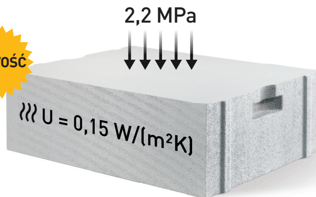
Grubość przegrody potrzebna do uzyskania współczynnika U \leq 0,20 \text{ W/(m}^2\text{K)} 1)
